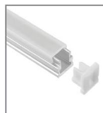
ACCE2083 IN0128AC PERFIL SOBREPUESTO 8x7.8x1000 mm INCLUYE TAPAS Y DIFUSOR
